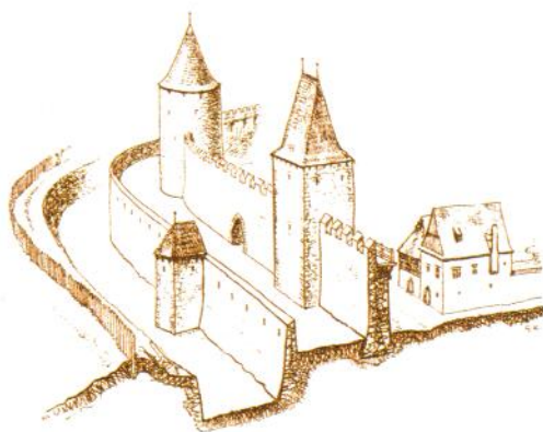
▲ Obr. 46 Hradební pásmo opevněného středověkého města. Za kúlovou palisádou na sypaném valu následuje příkop, dále vnější (parkánová) hradba, prostor mezi vnějším a vnitřním pásem hradeb (takzvaný parkán), vnitřní hradba rytizovaná věžemi či baštami a teprve poté vlastní městská zástavba
